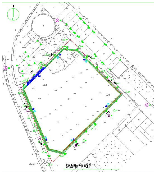
东莞市寮步莞樟路保障性住房项目基坑支护设计方案（基坑监测平面布置图）
